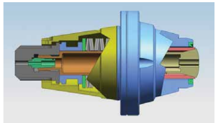
Patentierter Flexi-Chuck mit internen Federn
